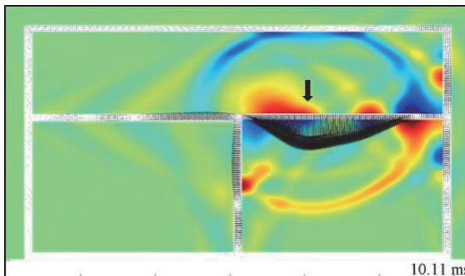
図中矢印位置を加振した場合の建築躯体の振動と放射音の可視化結果
