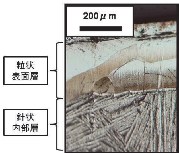
Ti-Ca合金の表面断層写真
