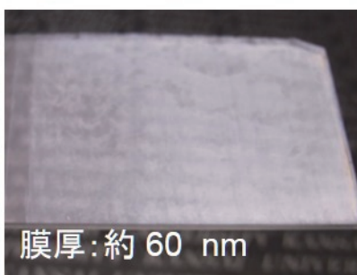
＜金属塩水溶液から作製された \text{SnO}_2 膜＞ 基材: 石英ガラス、熱処理: 700^\circ\text{C} \cdot 10 \text{ min}
