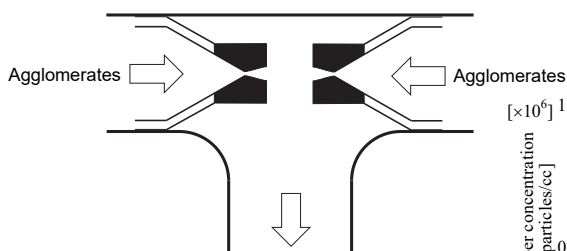
Fig. 1 凝集粒子同士を超音速流れの中で衝突させる
