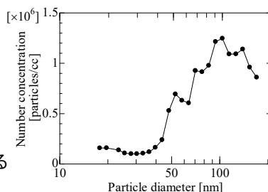
Fig. 2 衝突前の凝集粒子の粒径分布
