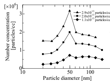
Fig. 3 分散化した50nmの非凝集粒子ピークを示す衝突後の凝集粒子粒径分布
